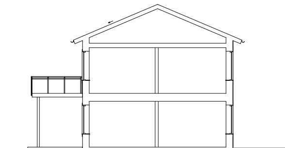
SEKTION A-A
