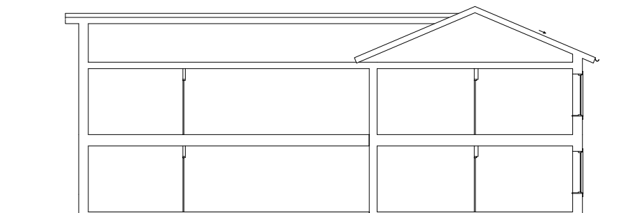
SEKTION C-C
