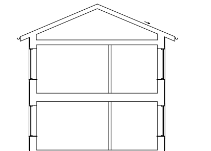
SEKTION B-B
